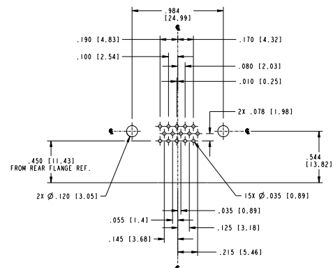
DEM15S (Receptacle)
