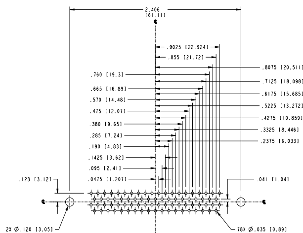
DDMM78S (Receptacle)
