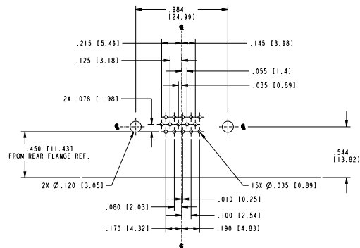
DEM15P (Plug)
